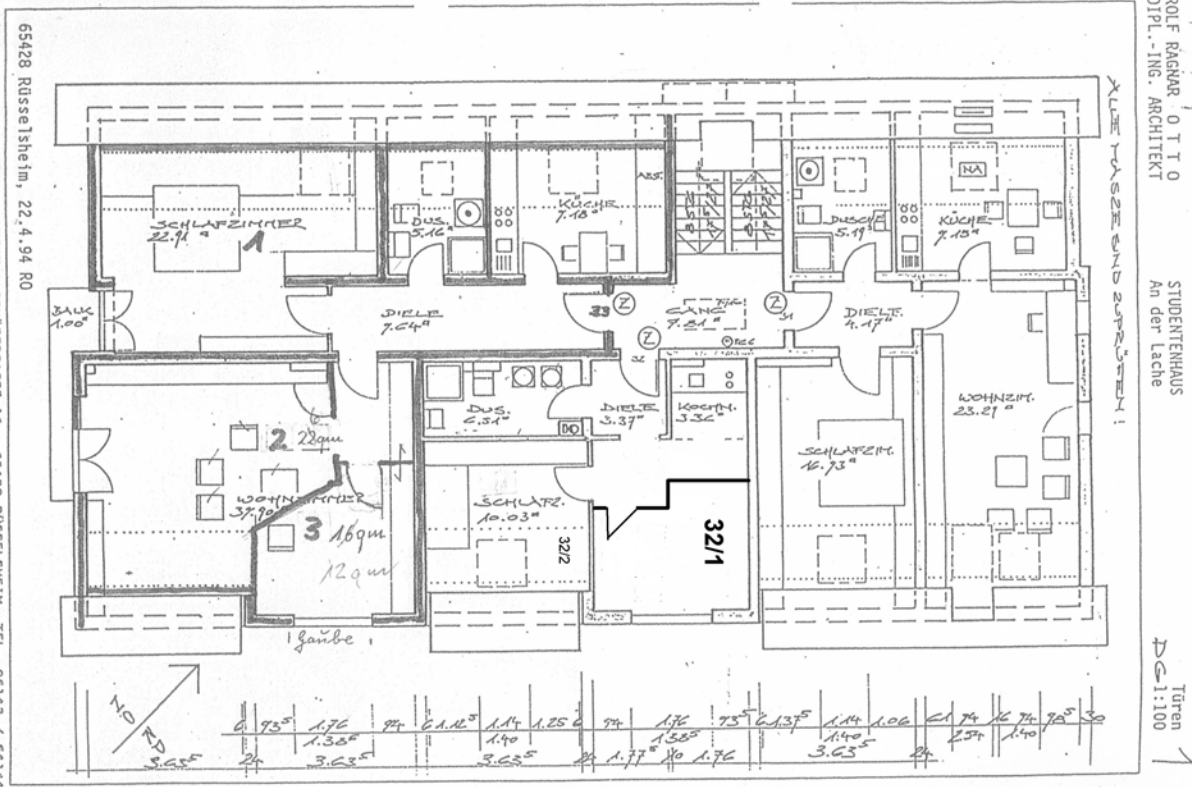
Plan 2er WG 32 und 3er WG 33
